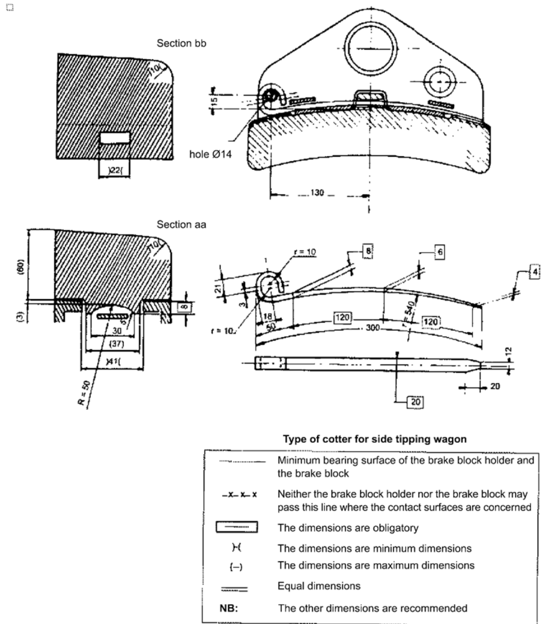
Fig part 1 U.K. I.10.3.2
