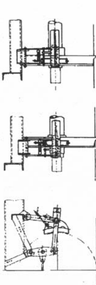
à titre indicatif : la bague n'est pas obligatoire zur Information: der Ring ist nicht verpflichtend purely indicative: ring not compulsory
