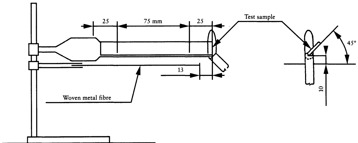
Test apparatus
